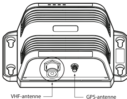
Figur 9 VHF-antennekontaktens posisjon
