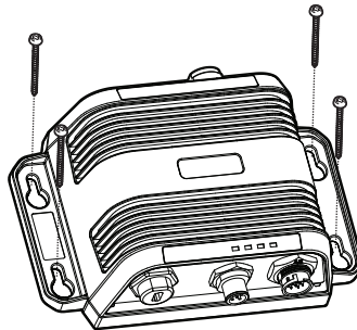
Figur 6 Montering av AIS-transceiveren
