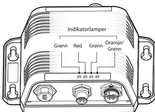
Figur 13 Plassering av indikator på AIS-transceiverenheten
